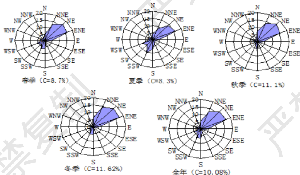
图 2-4 青阳各季及全年风向玫瑰图
