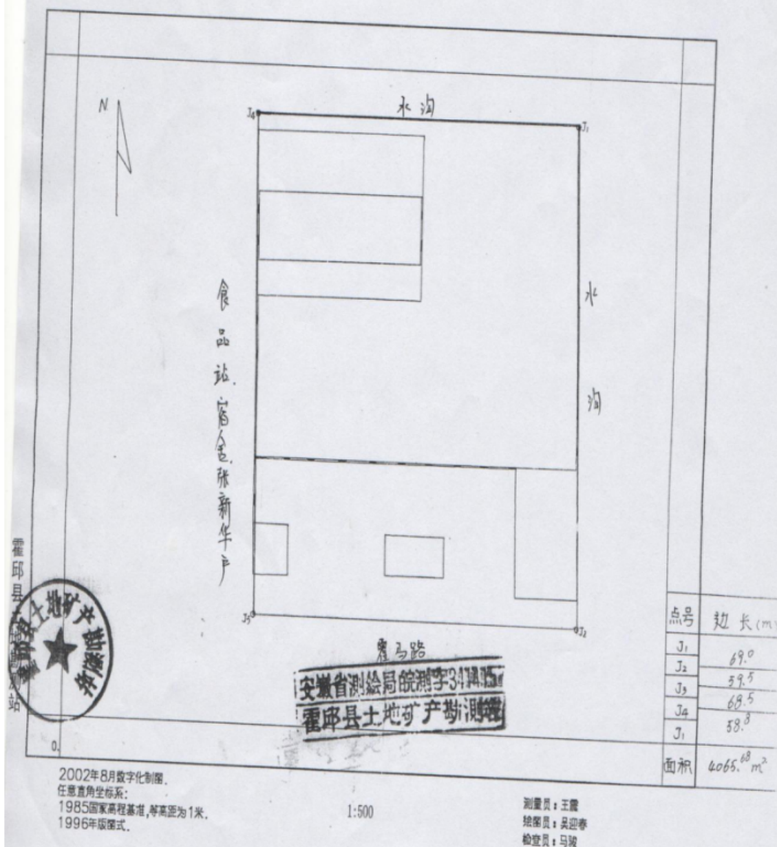
石油公司石店加油站地籍图
