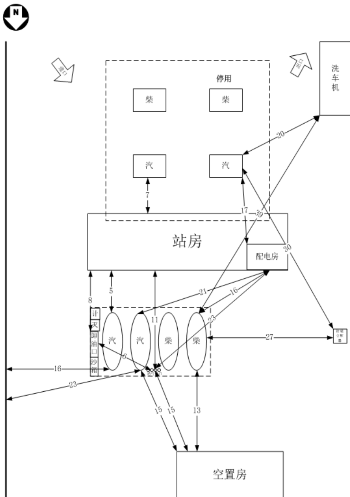
中石化霍邱石店加油站总平面布置示意图 标注单位：米
