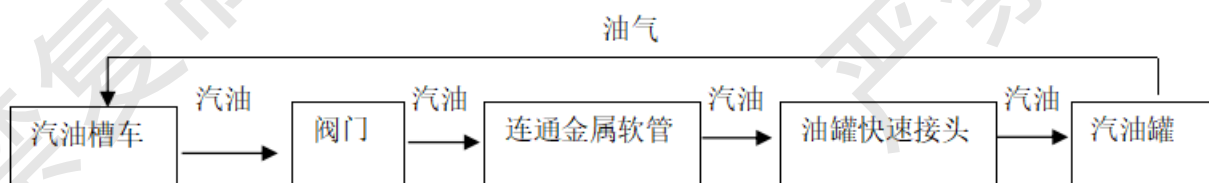
图 2-4 汽油卸油工艺流程
