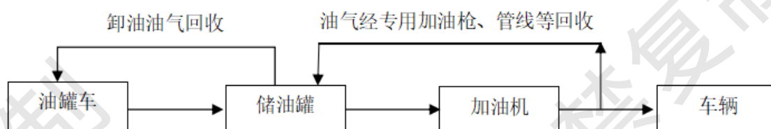
图 2-3 加油站工艺流程图
