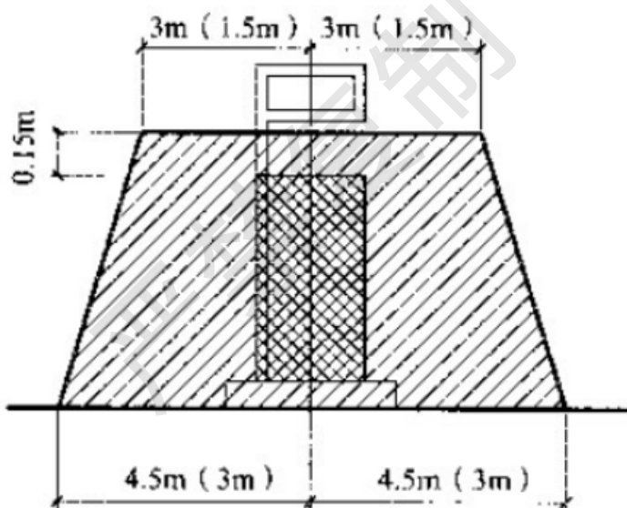
图 C.0.5 汽油加油机爆炸危险区域划分
