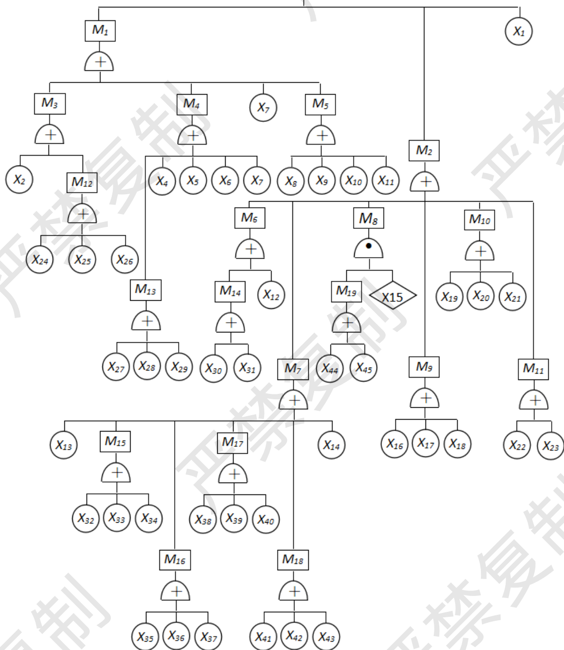
图 5-1 加油站事故树分析
