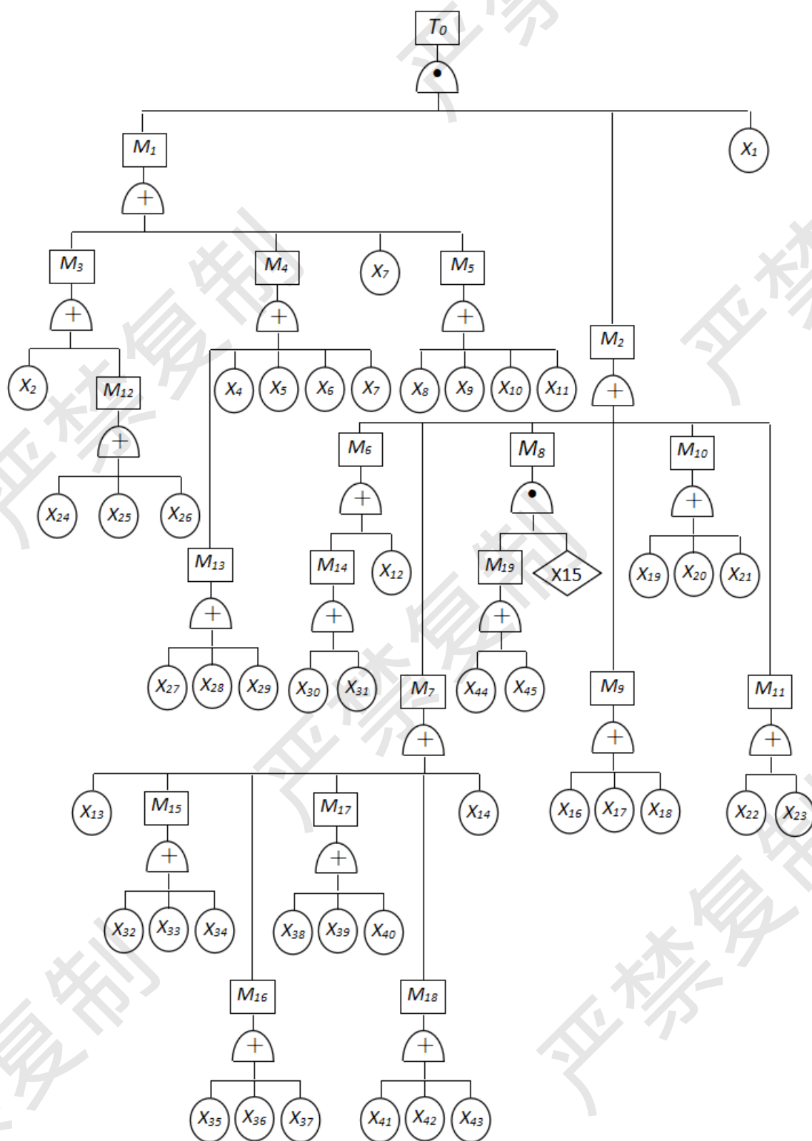
图 5-1 加油站事故树分析
