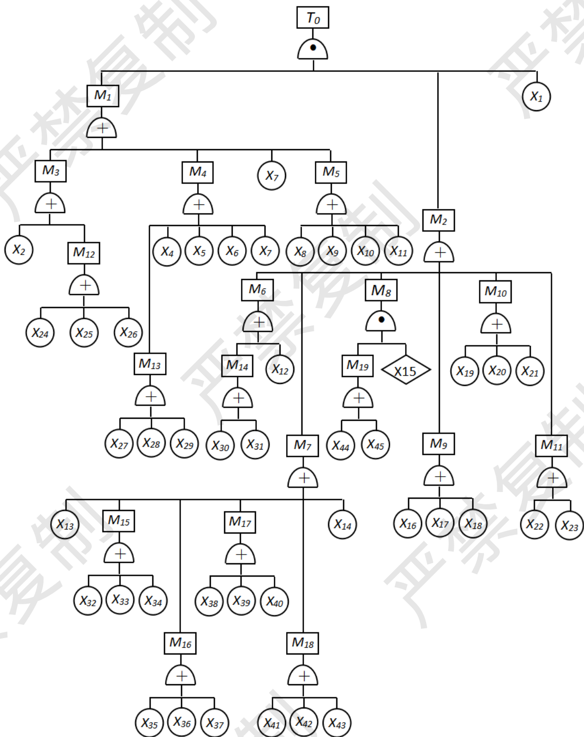
图 5-1 事故树分析
