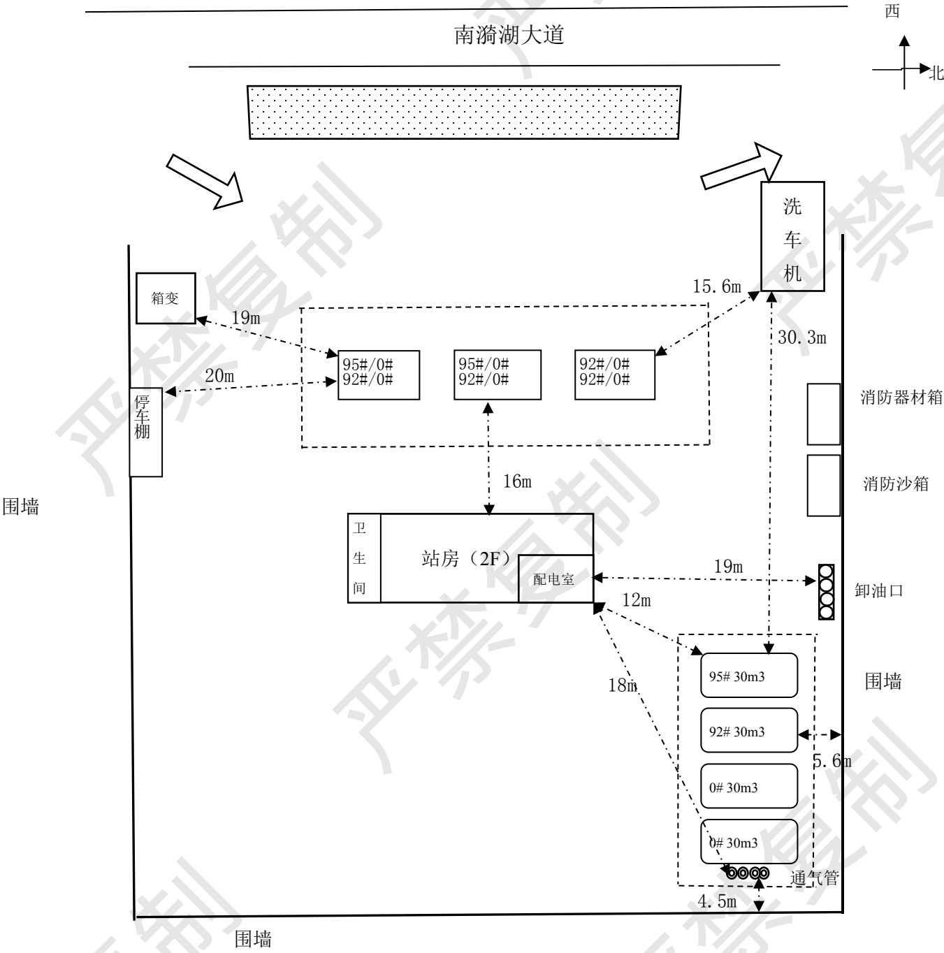
内部平面布置示意图（未标注安全间距见报告表 5-2）
