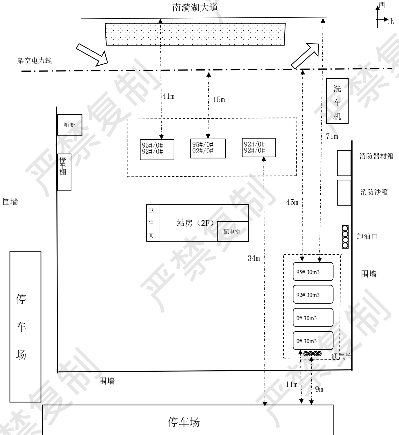
外部环境示意图（未标注安全间距见报告表 5-1）
