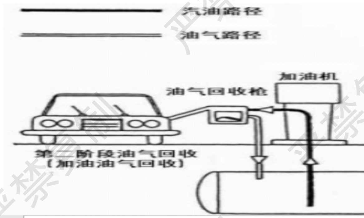
图 2-4 加油油气回收工艺流程图
