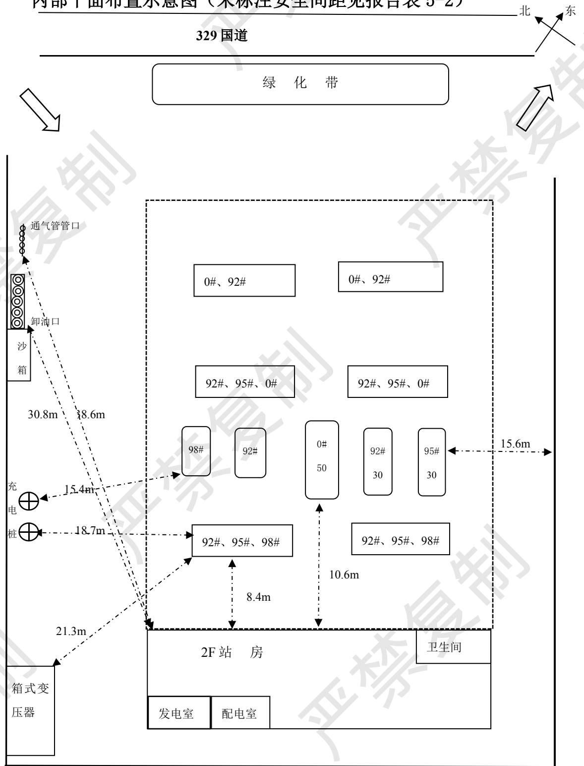
内部平面布置示意图（未标注安全间距见报告表 5-2）
