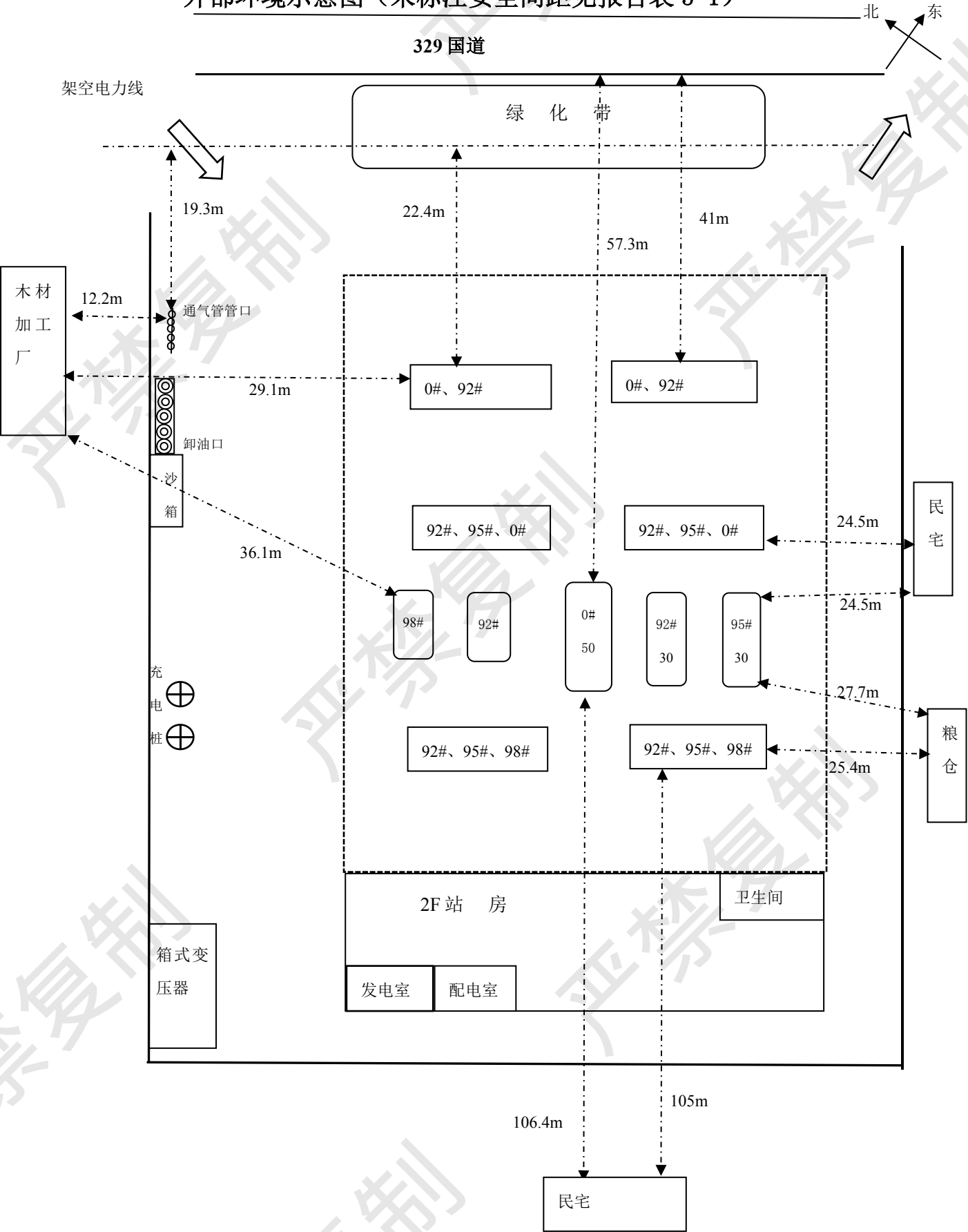
外部环境示意图（未标注安全间距见报告表 5-1）
