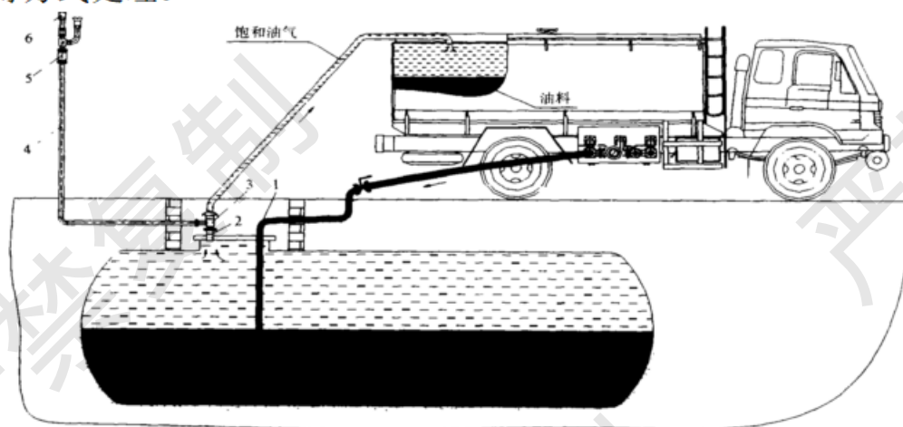
图 2-7 第一阶段油气回收系统示意图
