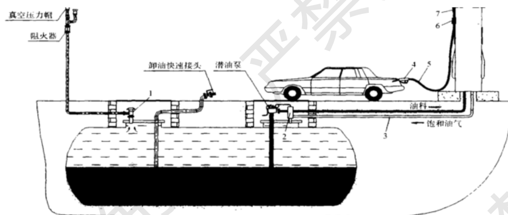
图 2-8 第二阶段油气回收系统示意图
