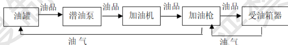
图 2-6 汽油加油工艺流程图
