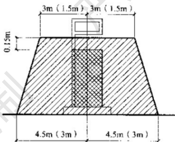
图 C.0.5 汽油加油机爆炸危险区域划分
