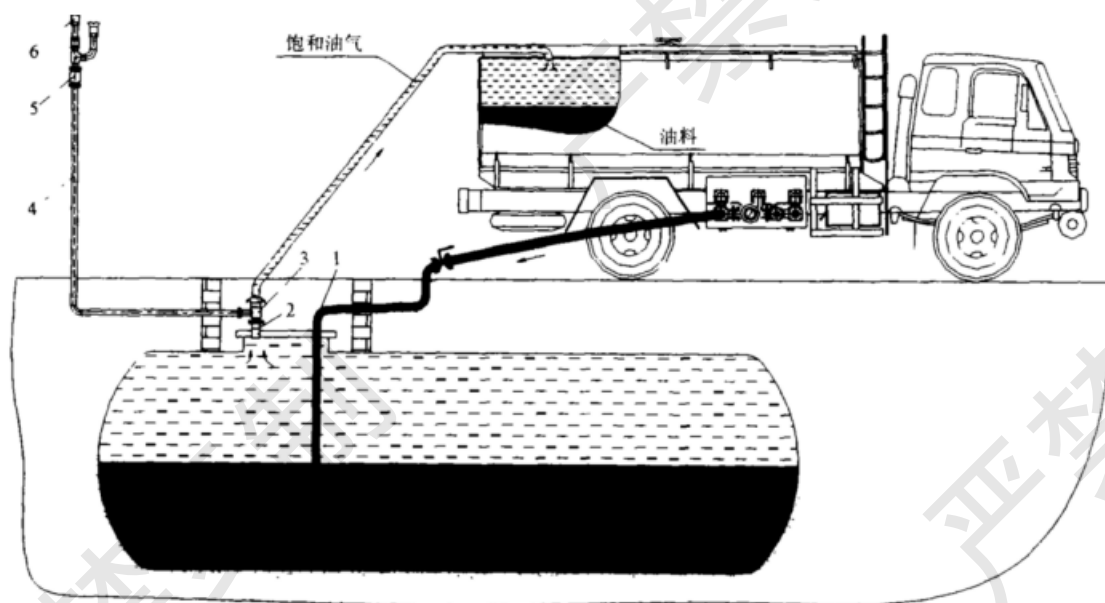
图 2-2 第一阶段油气回收系统示意图
