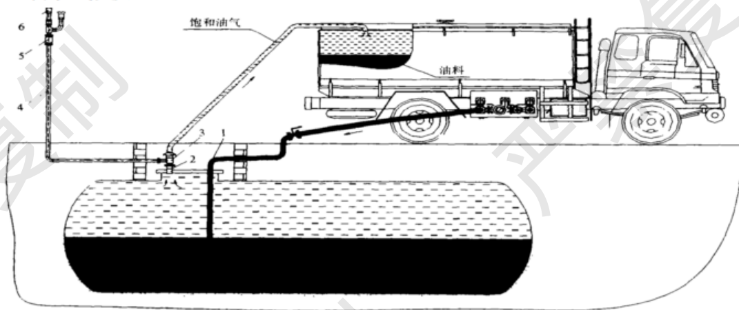
图 2-2 第一阶段油气回收系统示意图
