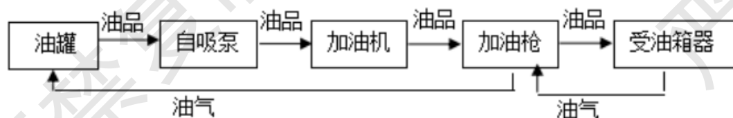
汽油加油工艺流程图
