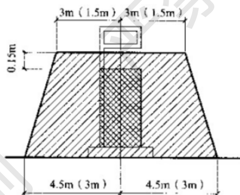
图 C.0.5 汽油加油机爆炸危险区域划分
