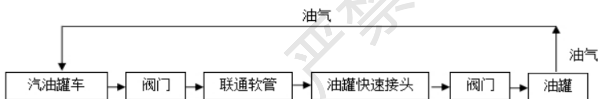
卸油工艺流程方块图
