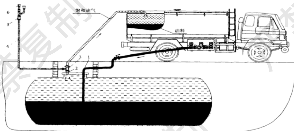
图 2-2 第一阶段油气回收系统示意图
