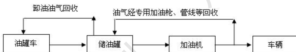
图 2.2 加油站工艺流程图
