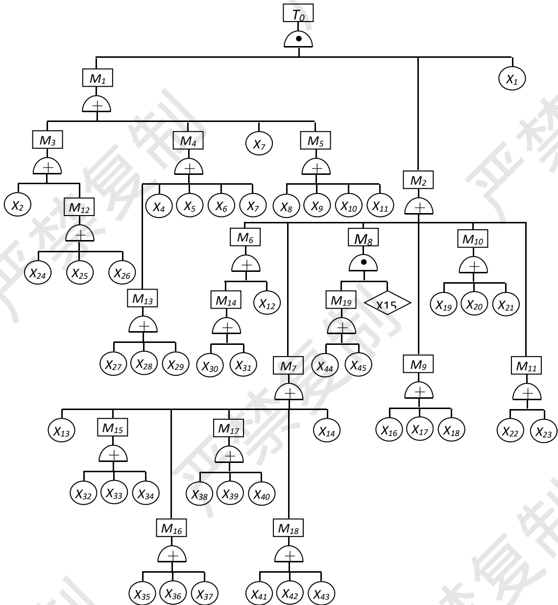
图 5-1 加油站事故树分析
