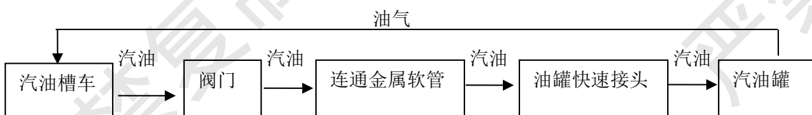
图 2-2 汽油卸油工艺流程
