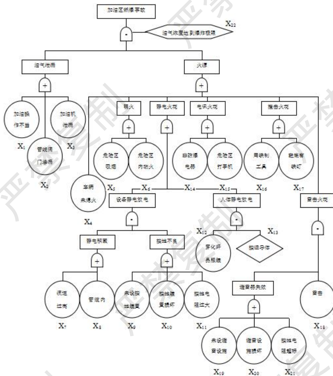
图 10-1 储罐区火灾、爆炸事故树
