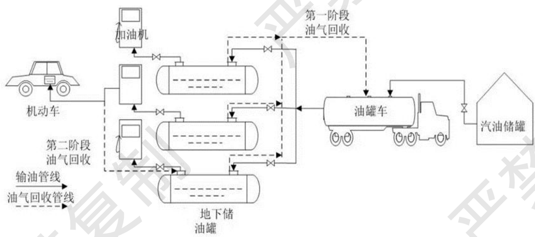
图 1-3 加油站油气回收系统示意图
