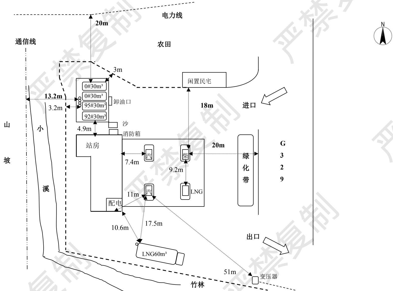
附件四 周边环境及平面布置示意图
