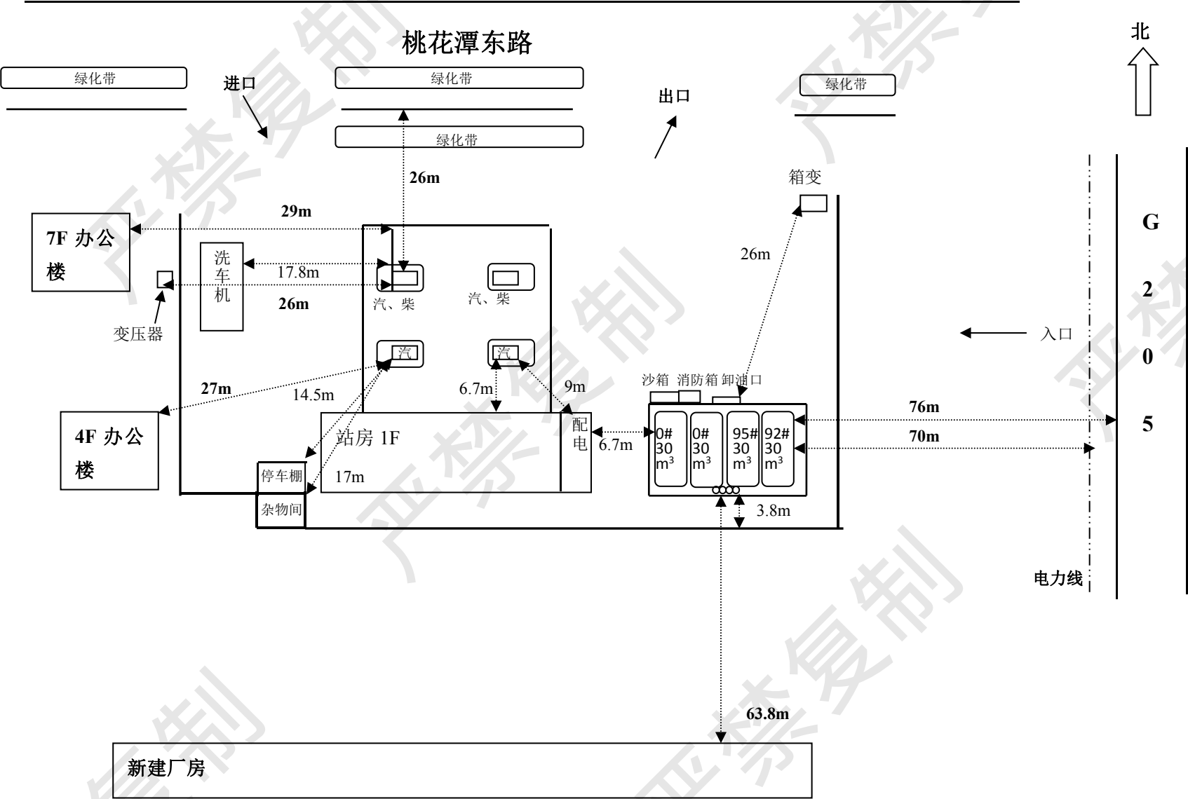
附件四 周边环境及平面布置示意图
