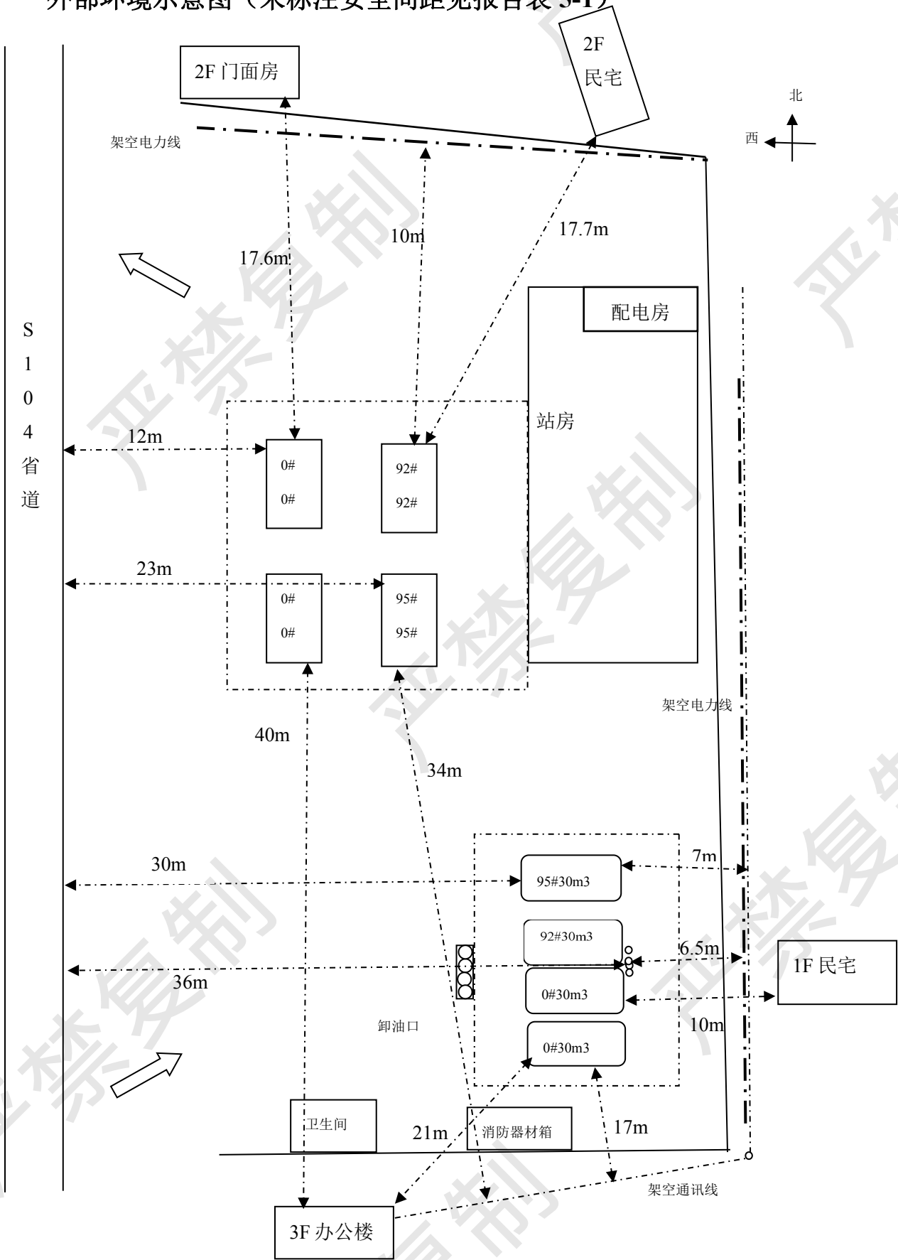
外部环境示意图（未标注安全间距见报告表 5-1）
