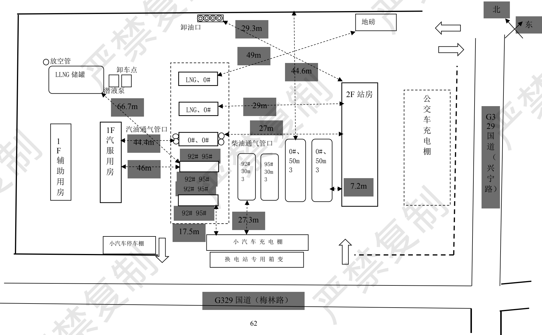
附件四 宁国市盛宁能源有限公司内部布置示意图
