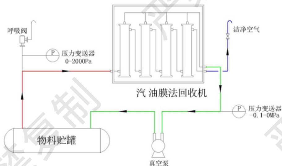
图 2-3 三次油气回收工艺流程图
