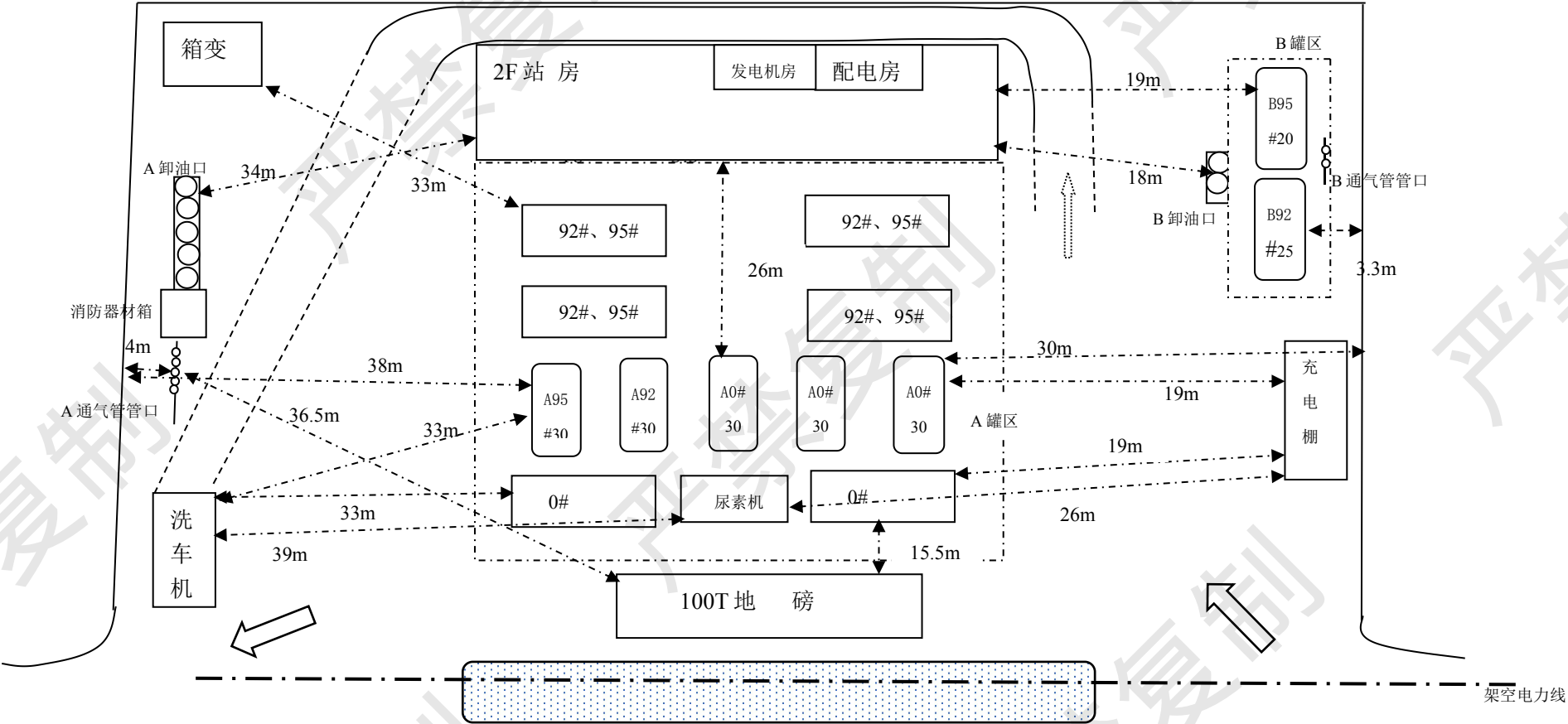
内部平面布置示意图（未标注安全间距见报告表 5-2）
