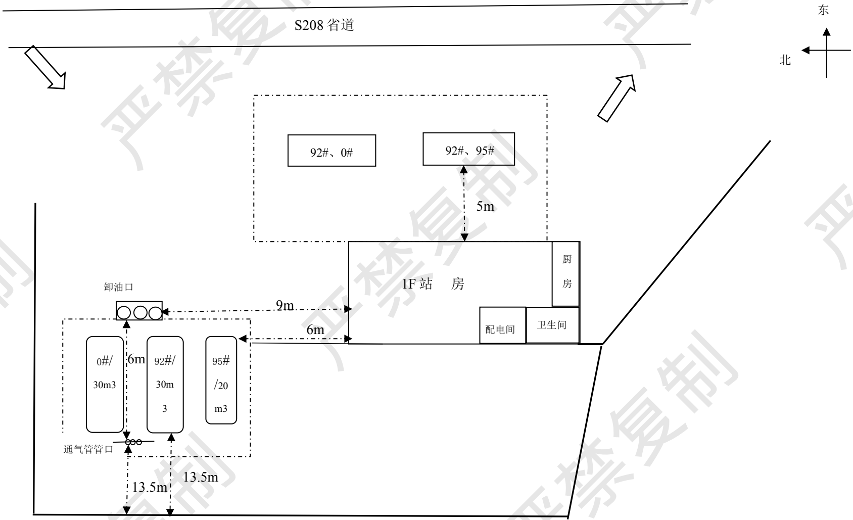
内部平面布置示意图（未标注安全间距见报告表 5-2）
