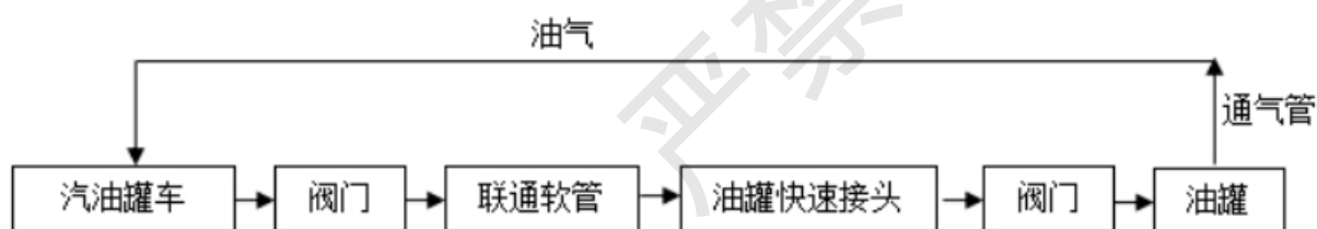
汽油卸油工艺流程方块图
