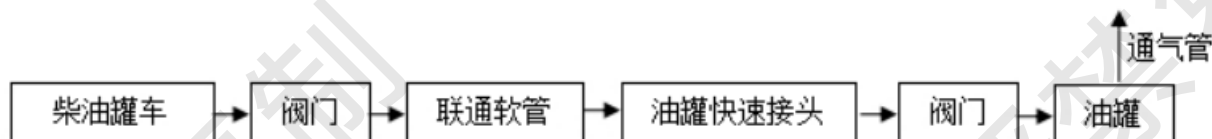
柴油卸油工艺流程方块图
