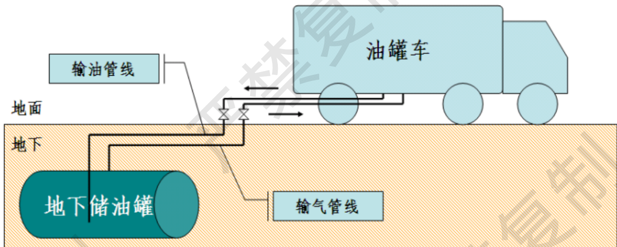
图 2-4 卸油油气回收工艺流程图
