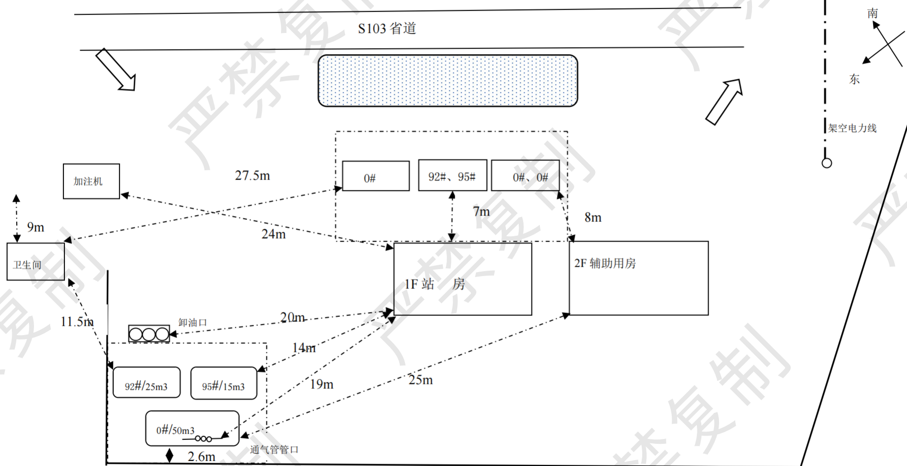
内部平面布置示意图（未标注安全间距见报告表 5-2）
