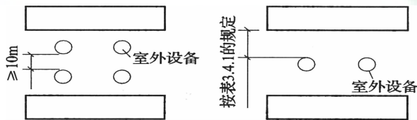
图 1 有室外设备时的防火间距
