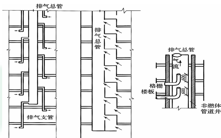
图1 排气管防止回流示意图
