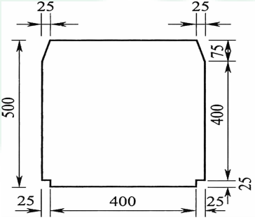
图 13 车行横通道的断面建筑限界(单位:cm)
