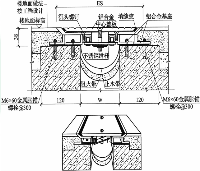
图 7 变形缝构造示意图
