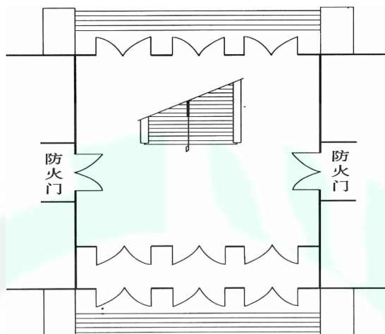
图5 扩大封闭楼梯间示意图
