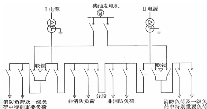
图 12 柴油发电机作为消防设备的备用电源的配电系统分组方案
