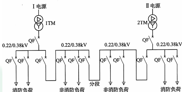
负荷不分组设计方案(二)
