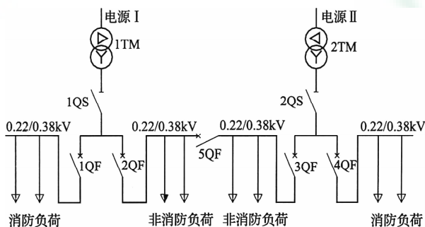
负荷分组设计方案(一)
