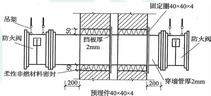
图 9 变形缝处的防火阀
