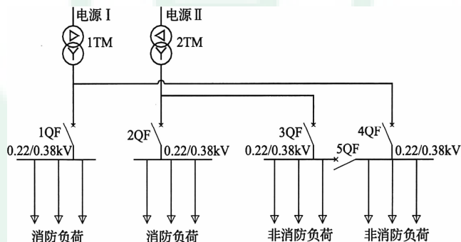
负荷分组设计方案(二)
