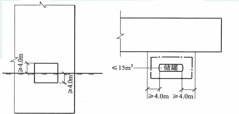
图 2 油罐面 4m 范围外墙设防火墙示意图
