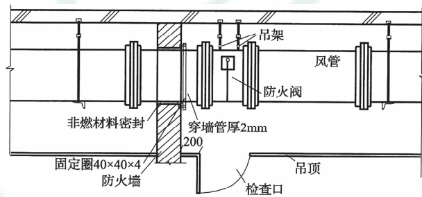
图 10 防火阀检修口设置示意图
